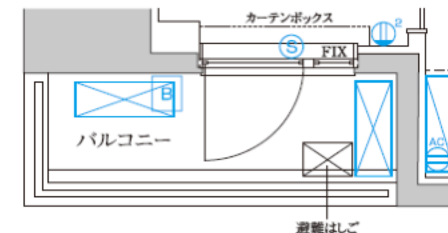
201号室部分図
