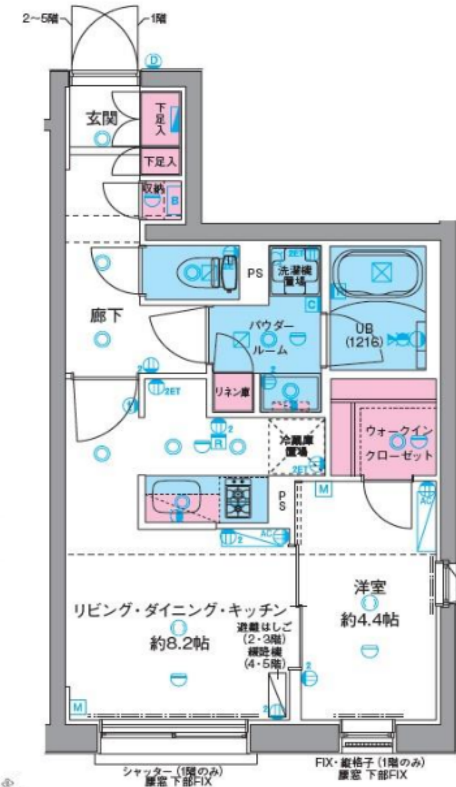
1階部分図
