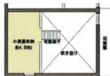
ロフト階平面図
