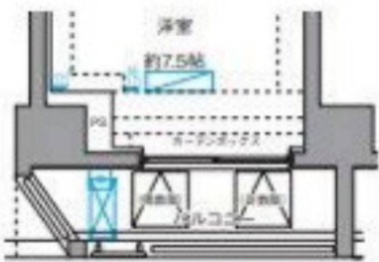
6階バルコニー図面
